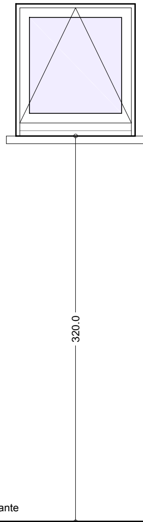
se.35 | finestrino bagno 2 dim. vano luce cm 62x68.5h superficie mq 0.42 movimento apertura a vasistas interna vetri 3+3/16/3+3 satinato
