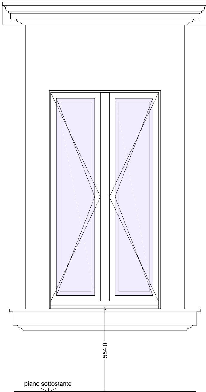
se.34 | finestra personale 2 dim. vano luce cm 99x193h superficie mq 1.91 movimento apertura alla francese vetri 3+3/16/3+3 trasparente scuri interni
