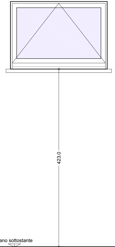
se.37 | finestra deposito dim. vano luce cm 109x76h superficie mq 0.83 movimento apertura a vasistas interna vetri 3+3/16/3+3 trasparente
